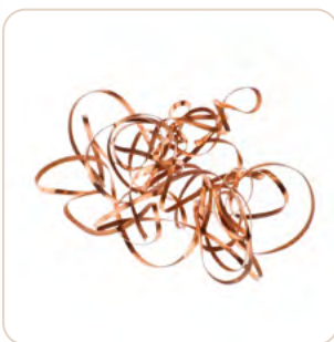
Werkstoff CuHCP: Langspanbildung hemmt den Arbeitsablauf beim Drehen.
