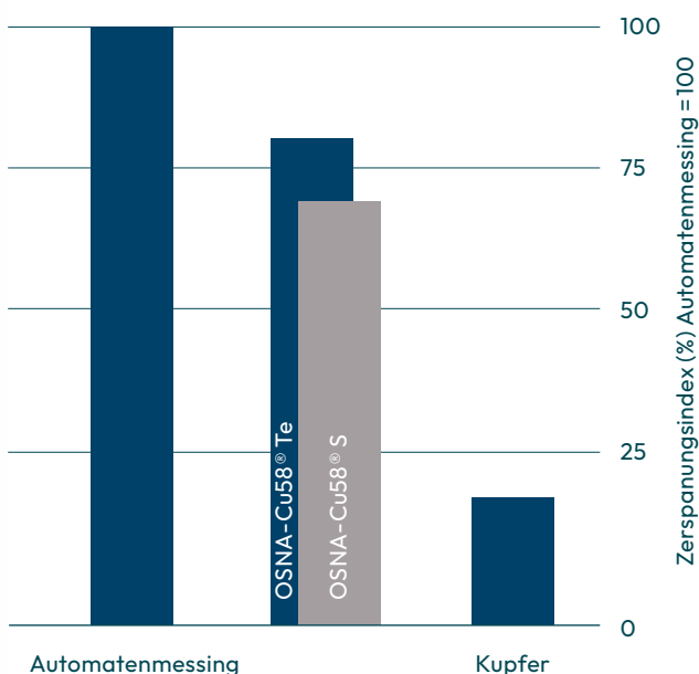
Zerspanungsindex von Automatenmessing OSNA-Cu58® und Kupfer
